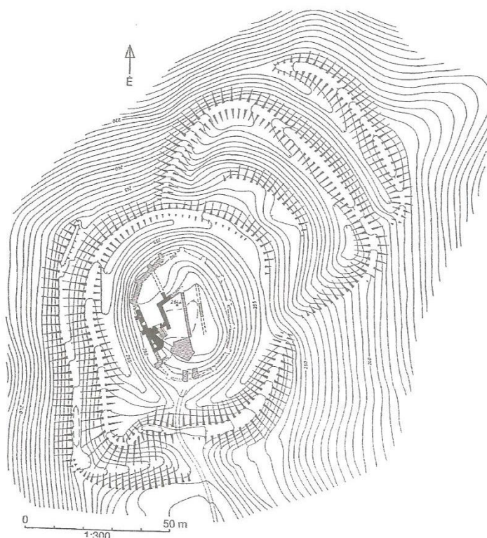
1. Kereki, Fehérkő vár. 1994. Felmérés és rajz: Nováki Gyula
