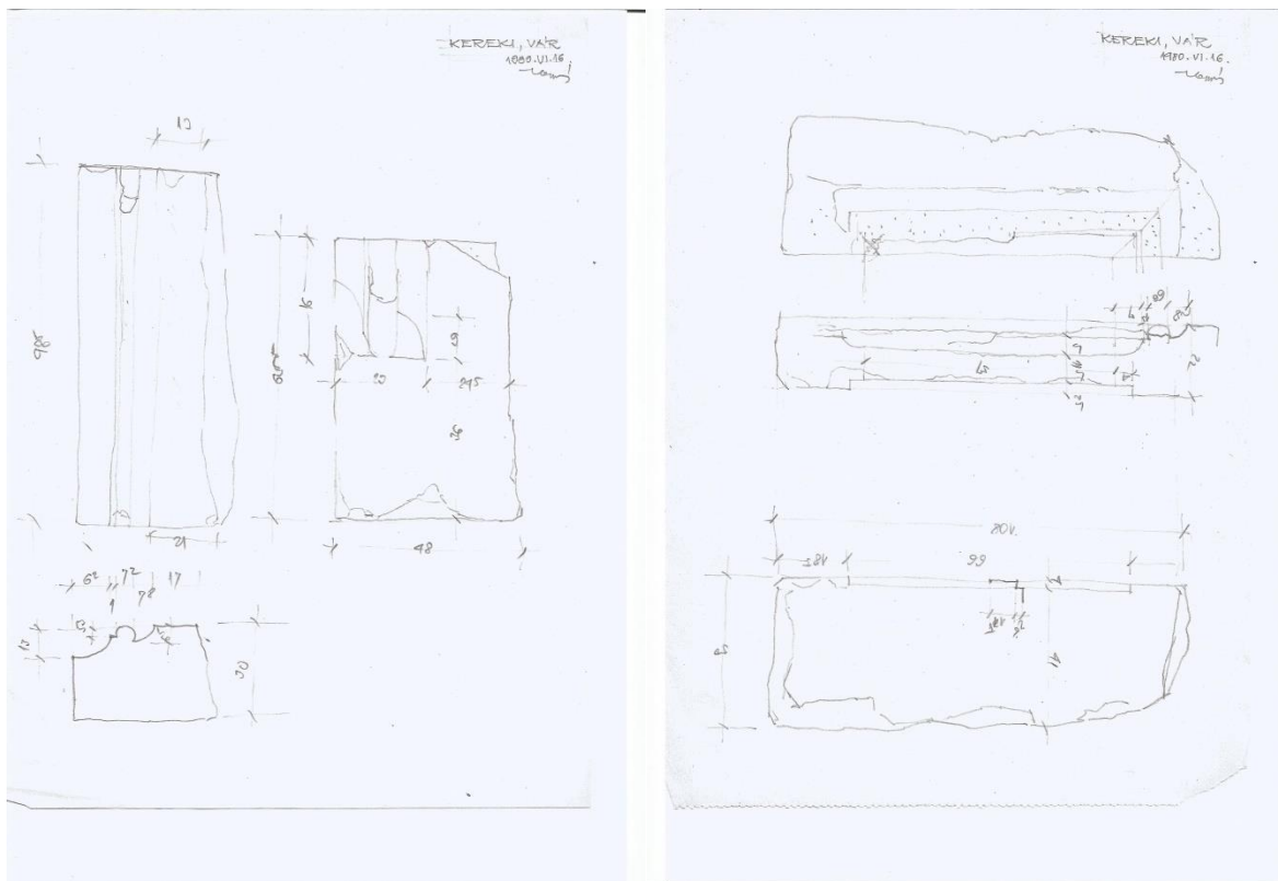
Ajtó szárkövek (2 db) és ablak szemöldökkő felmérése – Koppány Tibor 1980
