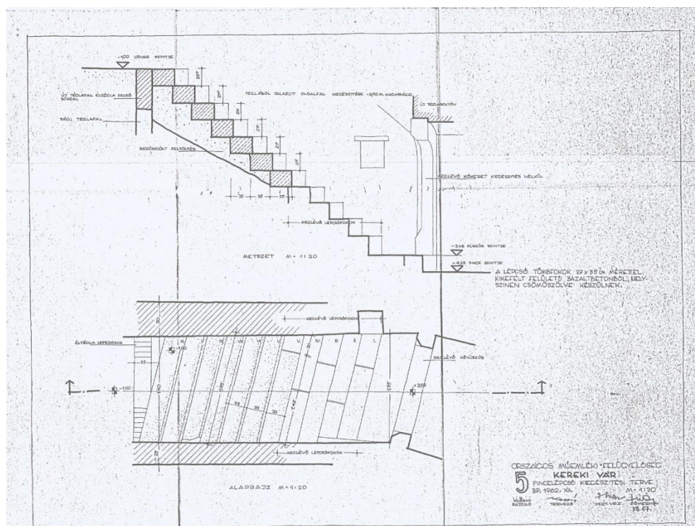
Pincelépcső – felmérés és terv
